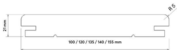
Lame face lisse fixation invisible B-Fix°
