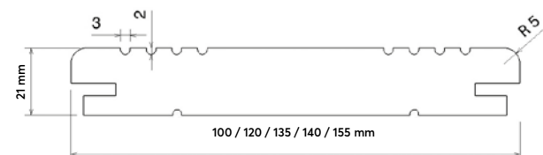
Lame face rainurée fixation invisible B-Fix°
