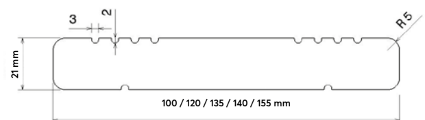
Lame face rainurée fixation traditionnelle
