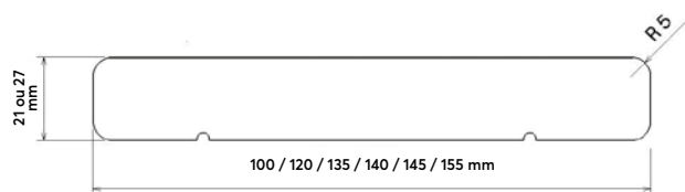
Lame face lisse fixation traditionnelle
