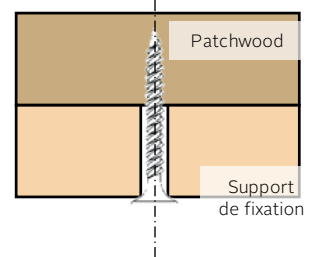
Fixation par vissage
