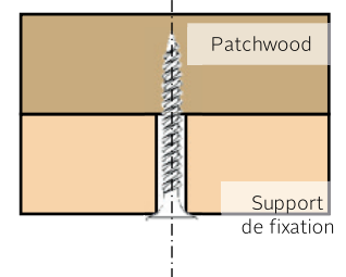
Fixation par vissage
